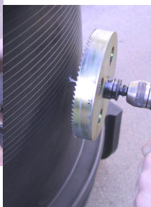
Bušenje rupice \phi 6 mm i . . .
